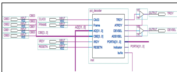
Fig. 11. Bloque del protocolo PCI.
