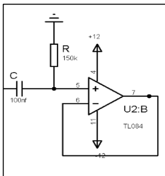
Fig.7. Filtro pasa altas de primer orden.
