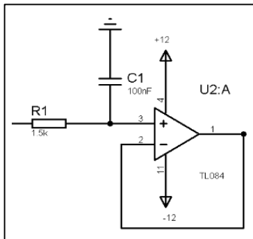
Fig.6. Filtro pasa bajas de primer orden
