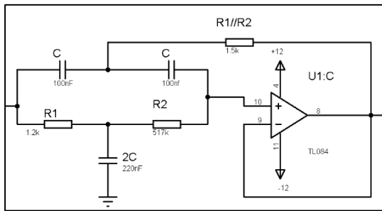
Fig.5. Filtro de rechazo de banda de estructura VCVS.
