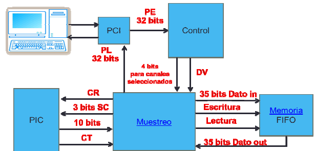
Fig. 12. Bloque de control de flujo de datos.
