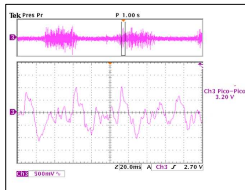
Fig.13. Señal mioeléctrica obtenida en las pruebas experimentales.
