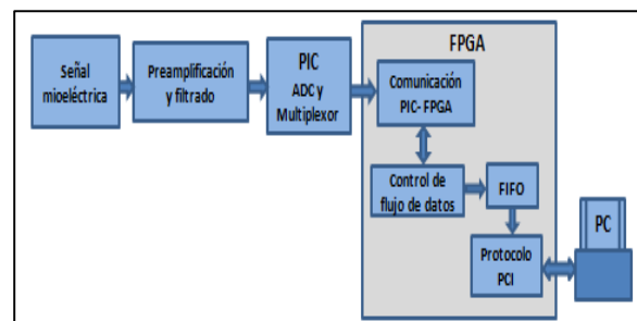
Fig.2. Diagrama a bloques general.
