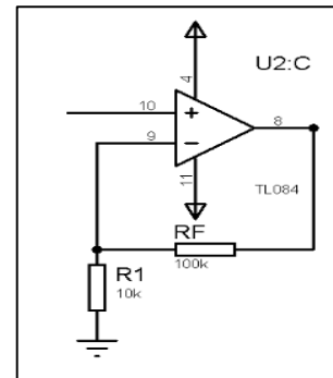
Fig.8. Amplificador no inversor.
