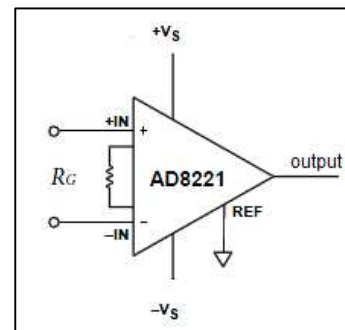
Fig.4. Amplificador de instrumentación AD8221.
