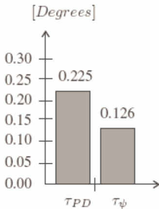
Figura 4. índice de Desempeño.
